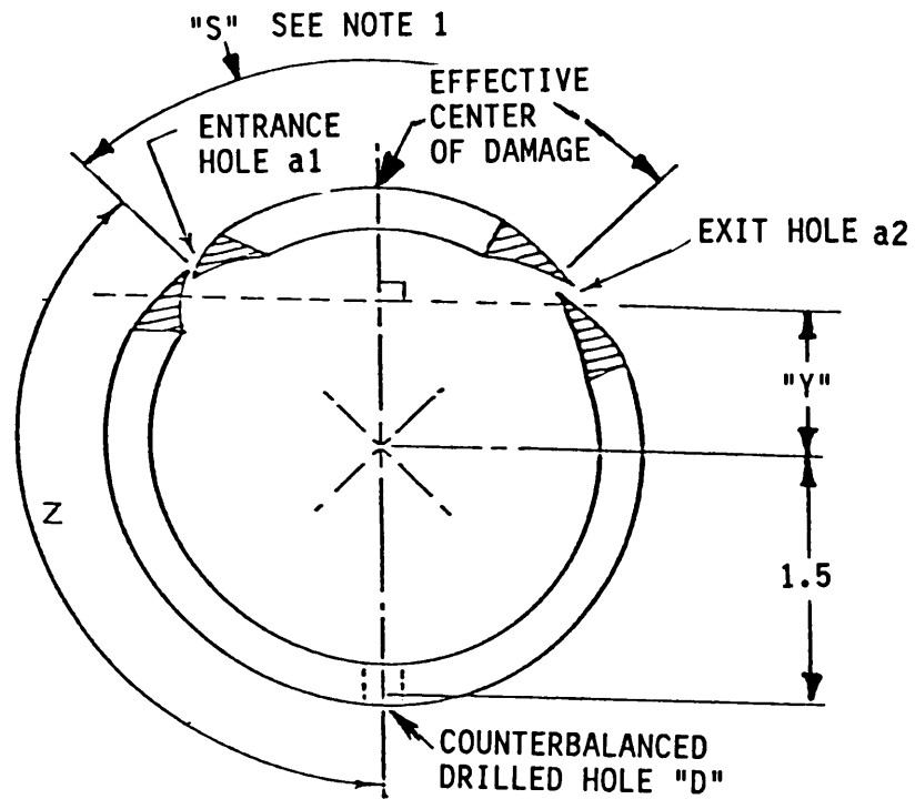
VIEW A-A
